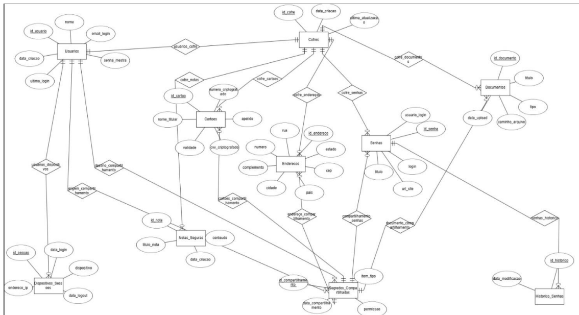
Diagrama Entidade-Relacionamento do sistema MeuCofre Seguro
